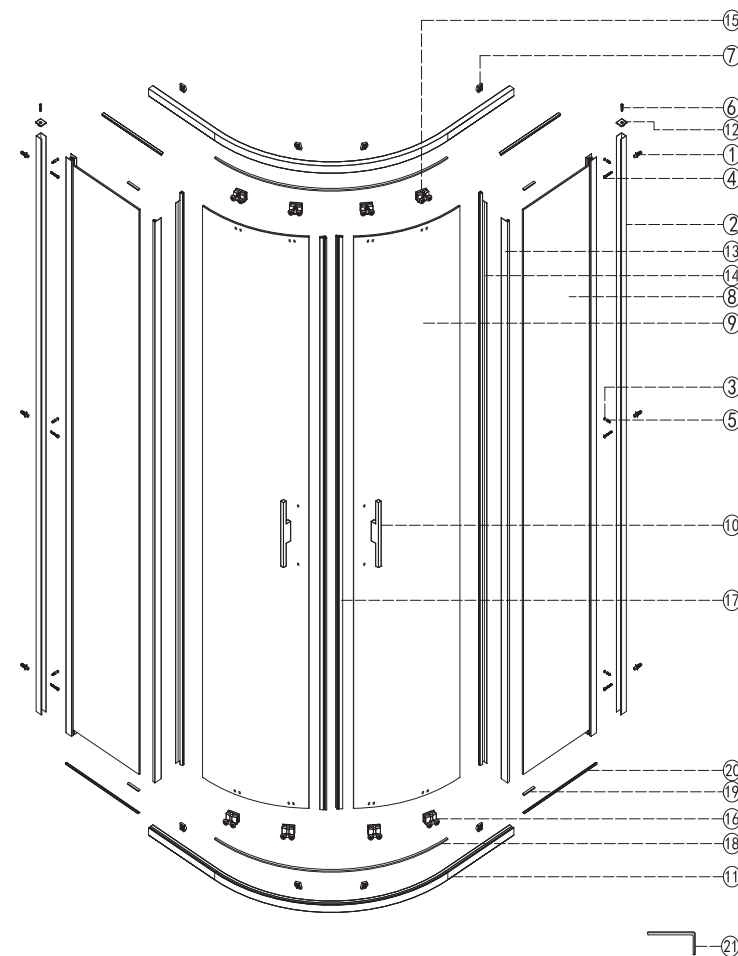
1. СХЕМА ИЗДЕЛИЯ
