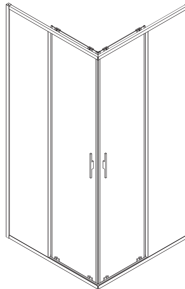
ДУШЕВОЕ ОГРАЖДЕНИЕ PRIORITY S
